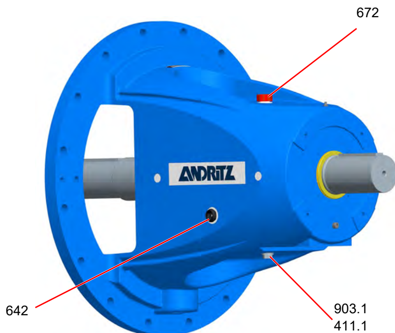
Рис. 29: Замена масла
