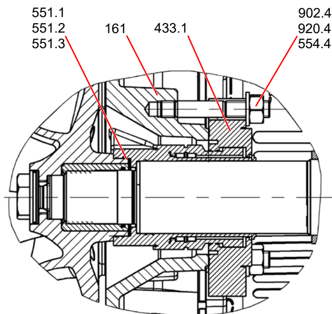
Рис. 33: Патронное уплотнение ANDRITZ BS24 – BS32
