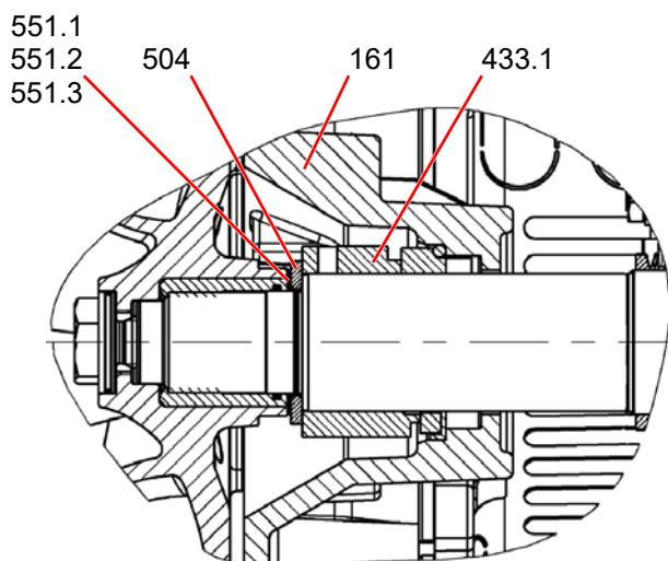
Рис. 16: Торцевое уплотнение простого действия (BS24 – BS32)
