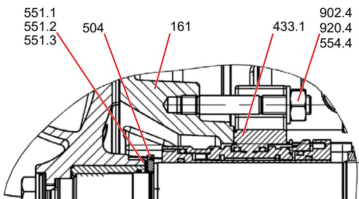
Рис. 39: Стандартное патронное уплотнение BS24 – BS32
