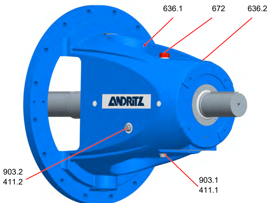
Рис. 28: Замена смазки
