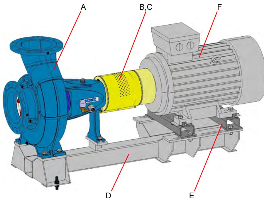
Рис. 6: Основные компоненты
