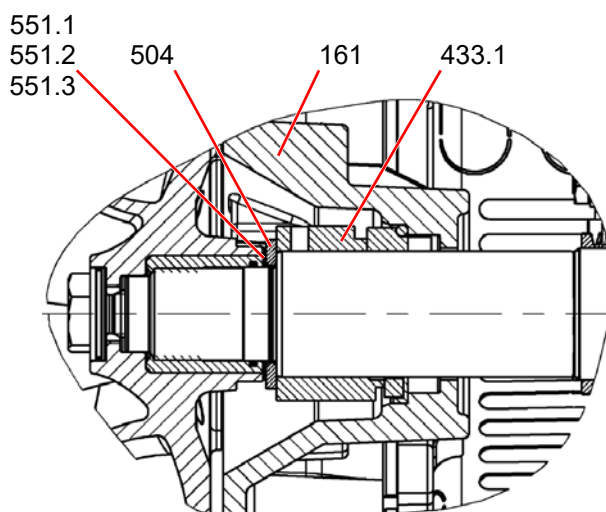
Рис. 37: Торцевое уплотнение BS24 - BS32
