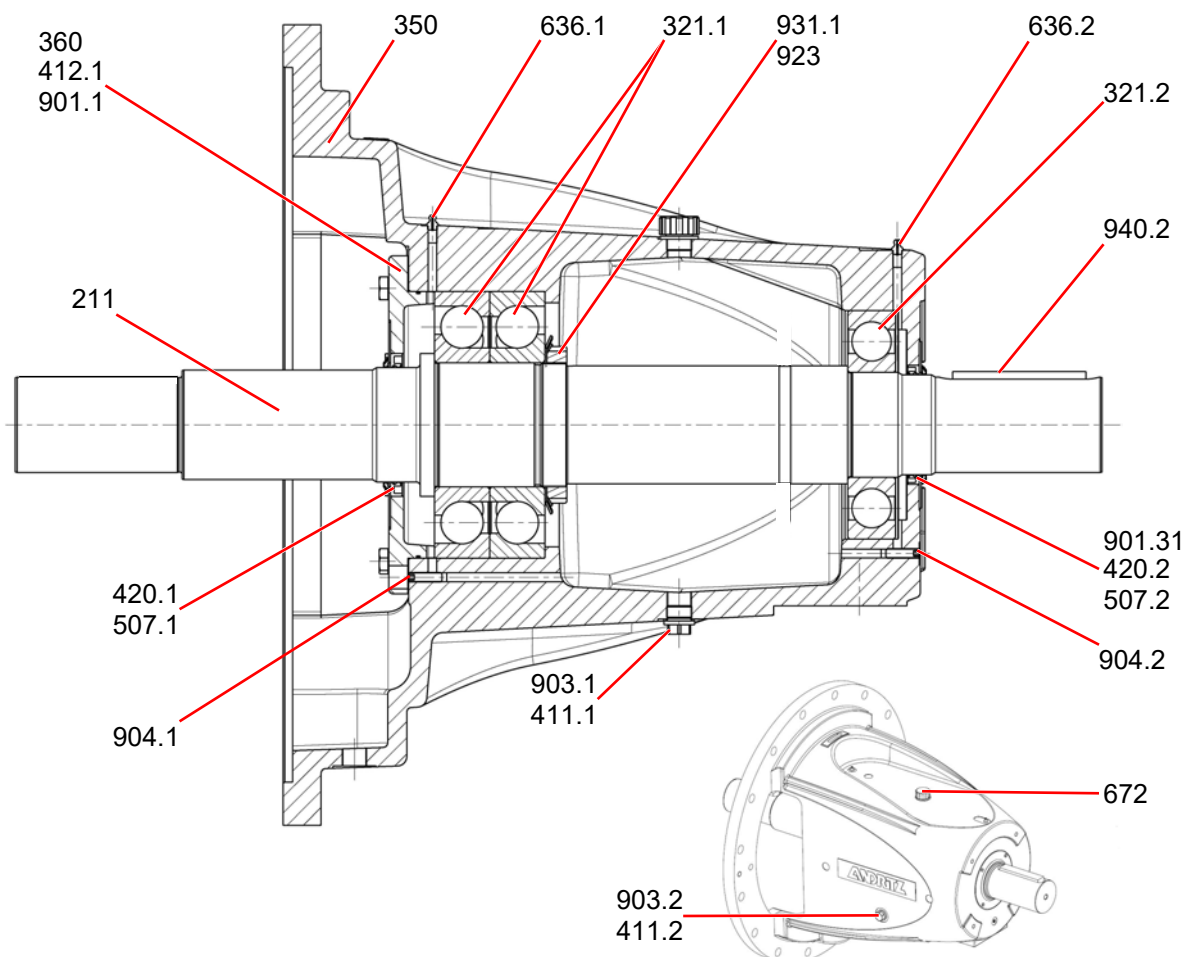
Рис. 9: Опора подшипников с консистентной смазкой
