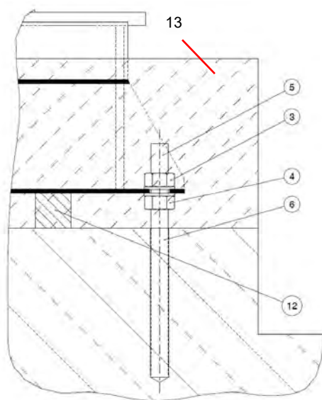
Рис. 26: Фундаментные работы
