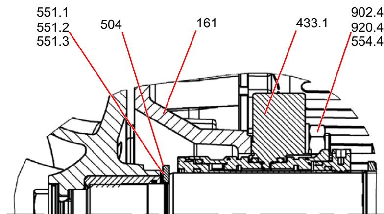
Рис. 41: Стандартное патронное уплотнение BS24 – BS32
