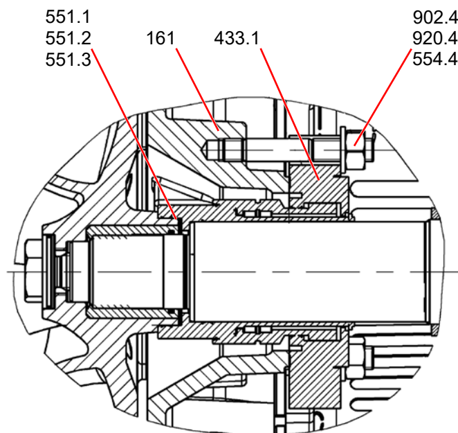
Рис. 12: Патронное уплотнение ANDRITZ (BS24 – BS32)
